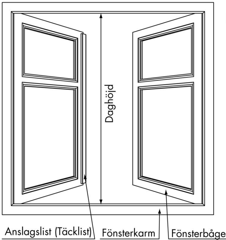
Utåtgående fönster med två mötesbågar
