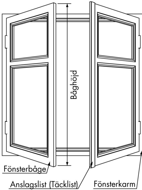
Inåtgående fönster med två mötesbågar
